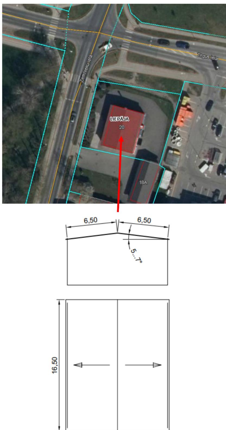
Attēls 1 Informatīva shēma paredzētās saules elektrostacijas ēkas jumtam KSS Nr. 4, Zemnieku ielā 20, Liepājā
