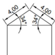
Attēls 3. Informatīva shēma paredzētās saules elektrostacijas ēkas jumtam Ventas ielā 11/17, Liepājā
